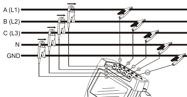
图 1. 分析仪与三相配电系统的连接
